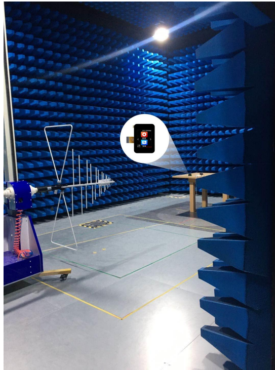
图 7-5 辐射测试图
