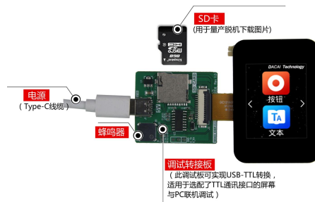
图 1-3 调试工具图
